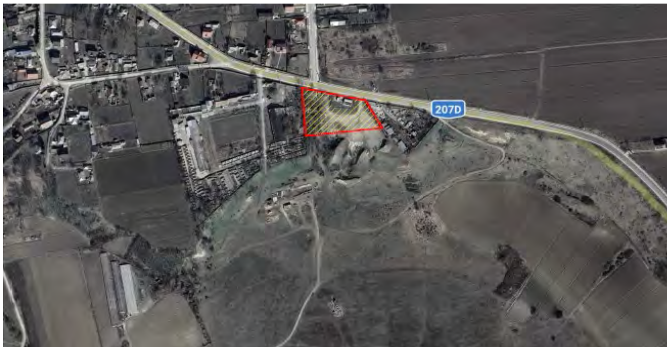
Fig. 1. Terenul propus pentru amplasare panouri fotovoltaice
